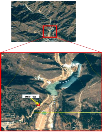
野外考察路线南段局部放大地形地貌图
